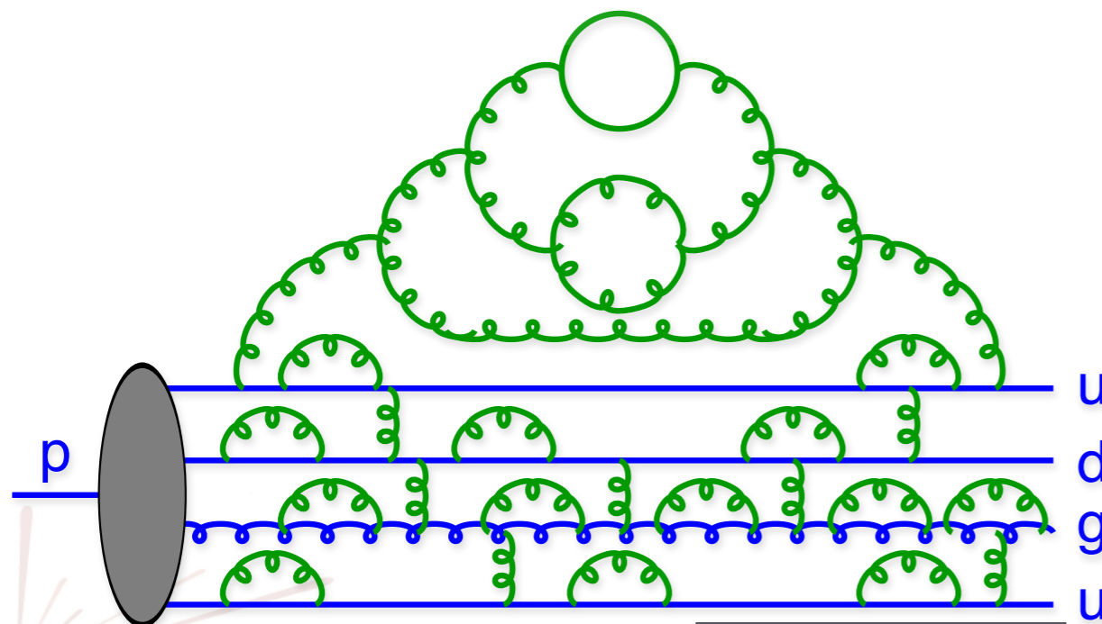
illustration by T. Sjöstrand
